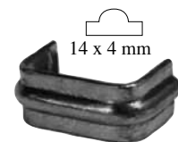
Art. 39/3 Fascetta di unione per 4 ferri Collar will accept 4 bars of 8 mm
