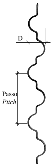
Art. 38/2 12 x 6 mm D 80 per mm 240 mm Passo - Pitch H 1600 mm
